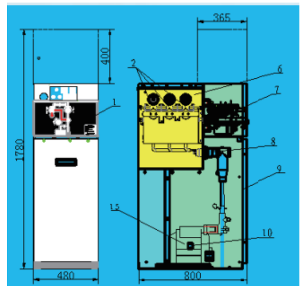
Ячейка с выключателем нагрузки и измерительным трансформатором напряжения (РТ)
