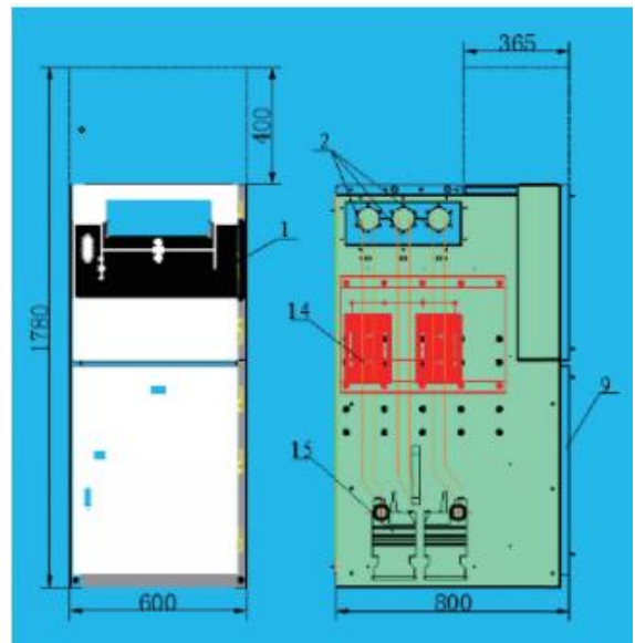
Ячейка с измерительными трансформаторами тока и напряжения (М)
